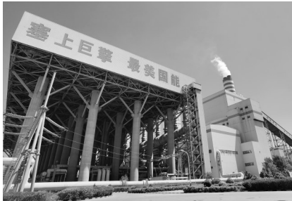
国能宁夏灵武发电有限公司建设的全球首套百万千瓦级空冷机组,改变靠水冷却传统技术,实现节水环保效益。
