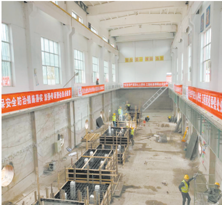
固海扩灌扬水更新改造工程8泵站施工现场。
