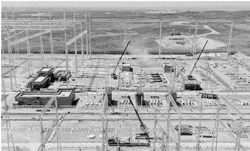
7月13日,在宁夏青山750千伏输变电工程、妙岭750千伏输变电工程、泉眼330千伏输变电工程、妙岭330千伏配电工程等近30余个施工现场,电网建设者们迎酷暑、战攻坚,积极应对夏季施工高峰考验。
